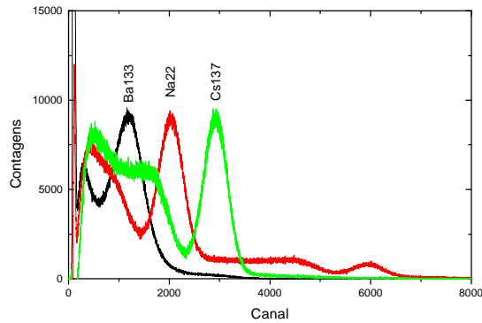
Figura 4. Espectros de energia obtidos com o mesmo conjunto detector, mas utilizando um monocanal comercial.
