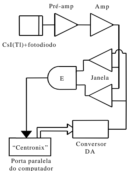
Figura 1. Diagrama de blocos do circuito eletrônico do espectrômetro.
