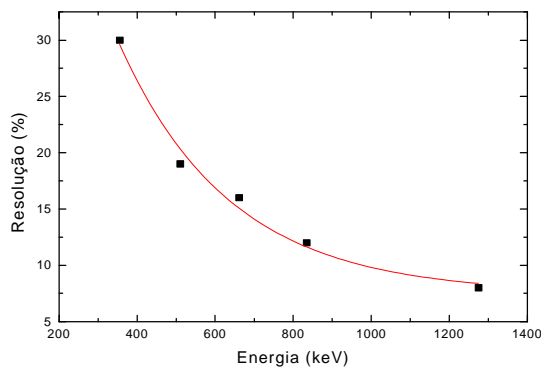
Figura 5. Resolução percentual em função da energia do raio gama incidente.
