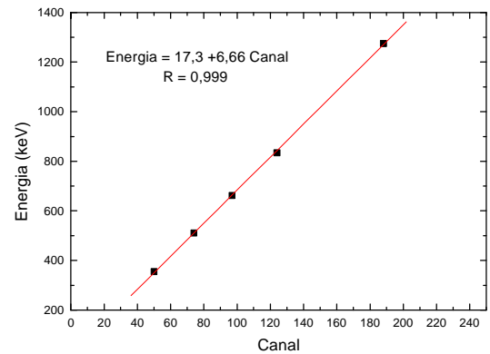
Figura 6. Linearidade da energia com o número de canal (Ganho do amplificador em 50%).
