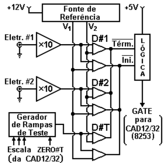
Figura 2. Módulo Eletrônico ActMASTER H01 (Diagrama Simplificado)
