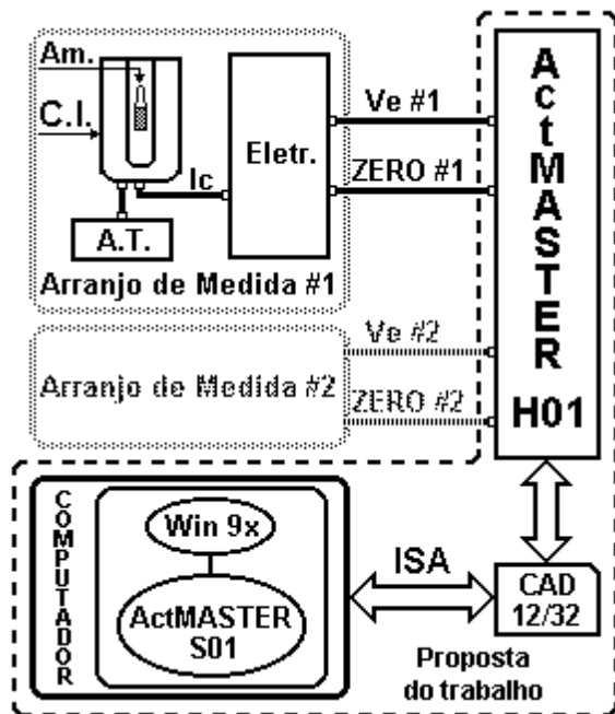
Figura 1. Diagrama em Blocos do Sistema de Medida
