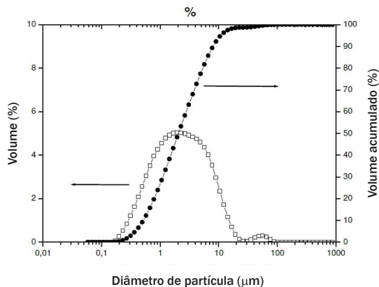
Gráfico 1 Distribuição do tamanho de partículas do cromito de lantânio dopado após duas horas de moagem.
