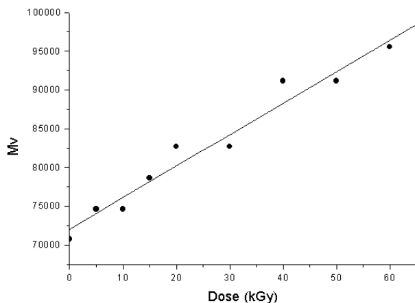
Figura 1 – Efeito da Dose de Irradiação na \overline{M}_v do PVAL
