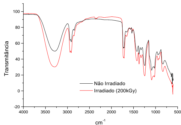
Figura 2 – Efeito da Irradiação na Estrutura Molecular do PVAL Estudado por FTIR
