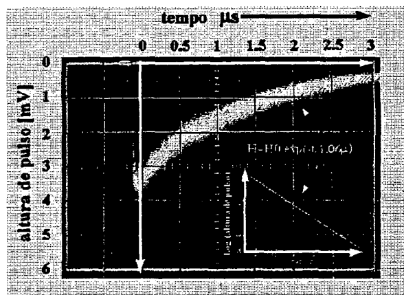
Figura 1. Sinal do Anodo da Fotomultiplicadora no Cristal Cintilador CsI(Tl).
