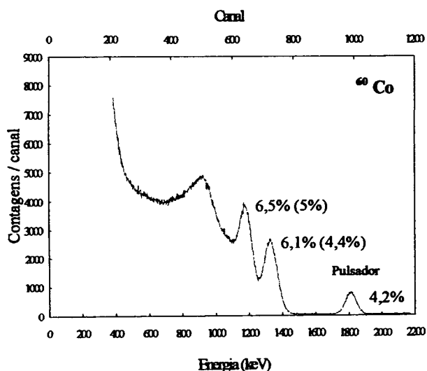
Figura 6. Espectro de Energia Obtido para a Radiação do ^{60}\text{Co} com o Cristal de CsI(Tl) Acoplado ao Fotodiodo.
