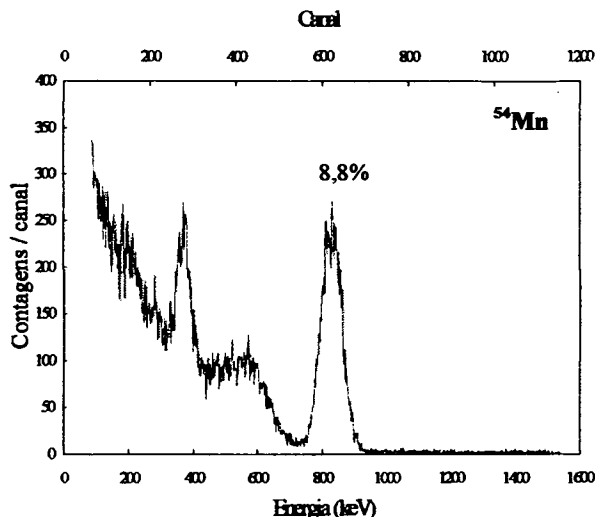
Figura 5. Espectro de Energia Obtido para a Radiação do ^{54}\text{Mn} com o Cristal de CsI(Tl) Acoplado à Fotomultiplicadora.
