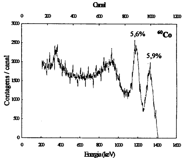
Figura 3. Espectro de Energia Obtido para a Radiação do ^{60}\text{Co} com o Cristal de CsI(Tl) Acoplado à Fotomultiplicadora.
