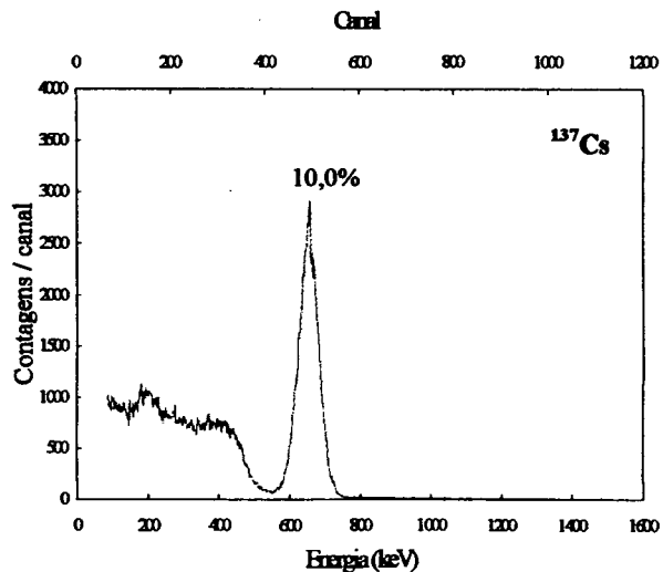
Figura 4. Espectro de Energia Obtido para a Radiação do ^{137}\text{Cs} com o Cristal de CsI(Tl) Acoplado à Fotomultiplicadora.
