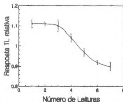
Figura 1 - Reprodutibilidade TL das pastilhas sem teflon.
