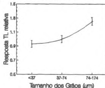
Figura 2 - Resposta TL para radiação gama em função do tamanho de grãos.
