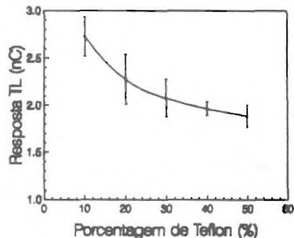
Figura 5 - Resposta TL para radiação gama em função da quantidade de teflon.
