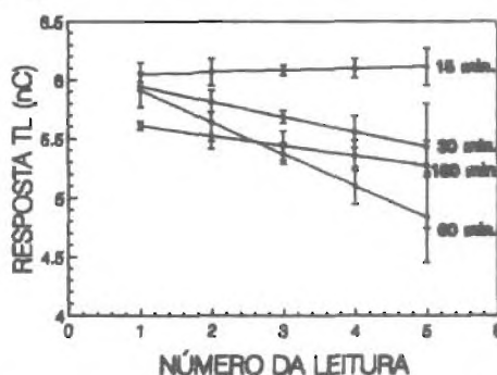
Figura 7 - Resposta TL em função do número de leituras para diferentes tratamentos térmicos.
