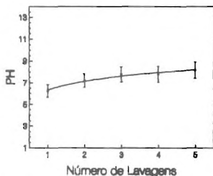
Figura 4 - PH da água utilizada para lavar o pó de MgB_4O_7:Dy em função do número de lavagens.
