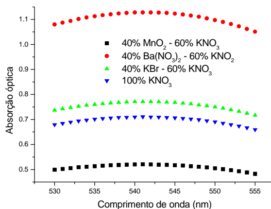
Figura 1. Espectro de Absorção. Intervalo de Comprimento de Onda entre 530 e 555 nm. Pastilhas de KNO 3 Puro e Misturas com Ba(NO 3 ) 2 , KBr e MnO 2 irradiadas com 300 kGy.
