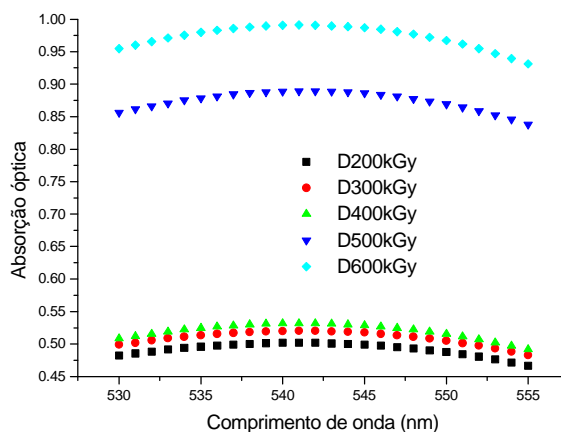
Figura 2. Espectro de Absorção de Pastilhas Confeccionadas com a Mistura 40% MnO 2 + 60% KNO 3 , Irradiadas com Doses entre 200 e 600 kGy.
