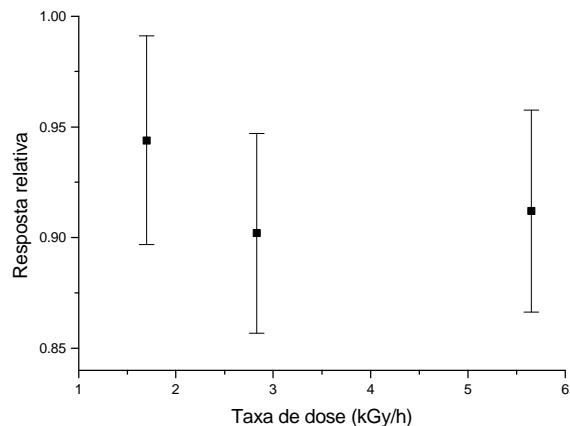
Figura 3. Variação da resposta com a taxa de dose para pastilhas produzidas com \text{KNO}_3 puro, irradiadas na fonte Gammacell com dose igual a 50 kGy.
