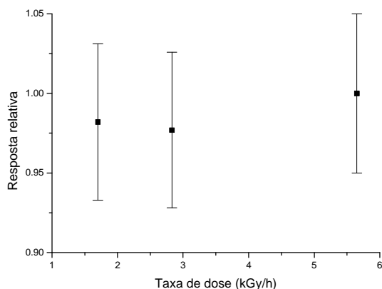
Figura 4. Variação da resposta com a taxa de dose para pastilhas produzidas com a mistura 40% \text{MnO}_2 + 60% \text{KNO}_3 , irradiadas na fonte Gammacell com dose igual a 50 kGy.
