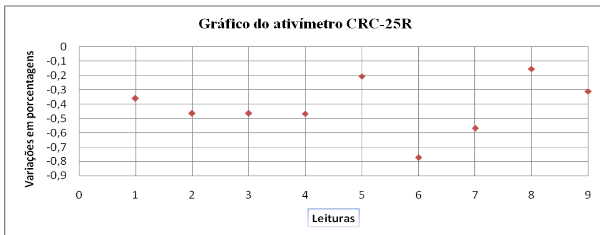
Figura 11. Resultado encontrado com o ativímetro CRC-25R.
