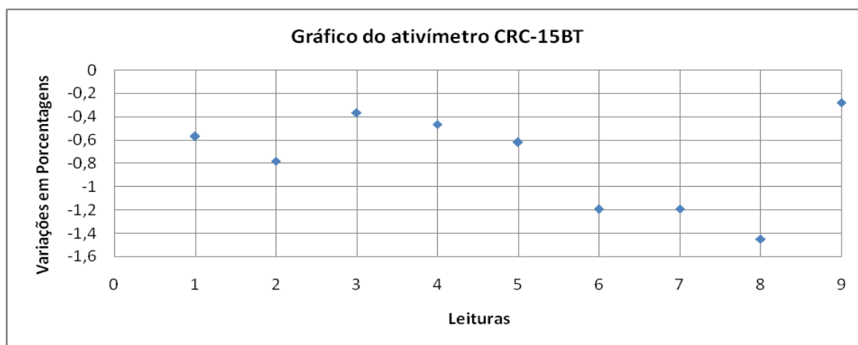
Figura 10. Resultado encontrado com o ativímetro CRC-15BT.
