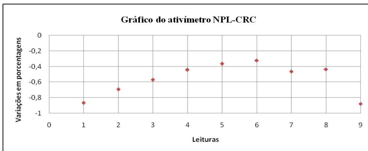
Figura 9. Resultado encontrado com o ativímetro NPL-CRC.
