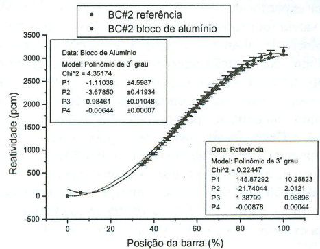
Figura 4. Curvas de Reatividade Integral da Barra BC#2: Referência e com Vazios Devidos a Presença do Bloco de Alumínio.
