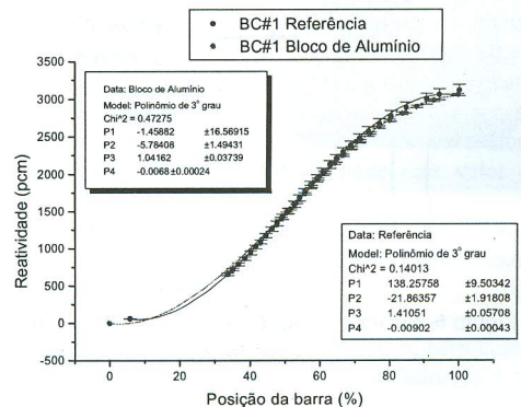
Figura 5. Curvas de Reatividade Integral da Barra BC#1: Referência e com Vazios Devidos a Presença do Bloco de Alumínio.
