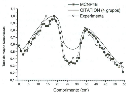
Figura 9. Distribuição da Taxa de Fissão na Vareta Experimental com a Presença do Bloco de Alumínio.
