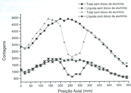
Figura 7. Distribuição da Taxa de Reação da Vareta Experimental.
