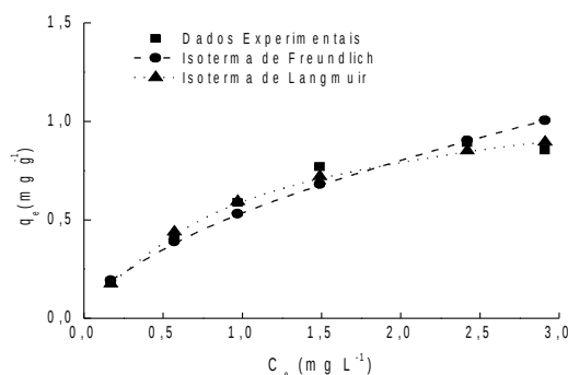
Figura 3. Isotherma de adsorção do RV sobre ZM-2 ( T = 25^\circ\text{C} ; \text{pH} = 5 ; t_{\text{agit}} = 360 \text{ min} )
