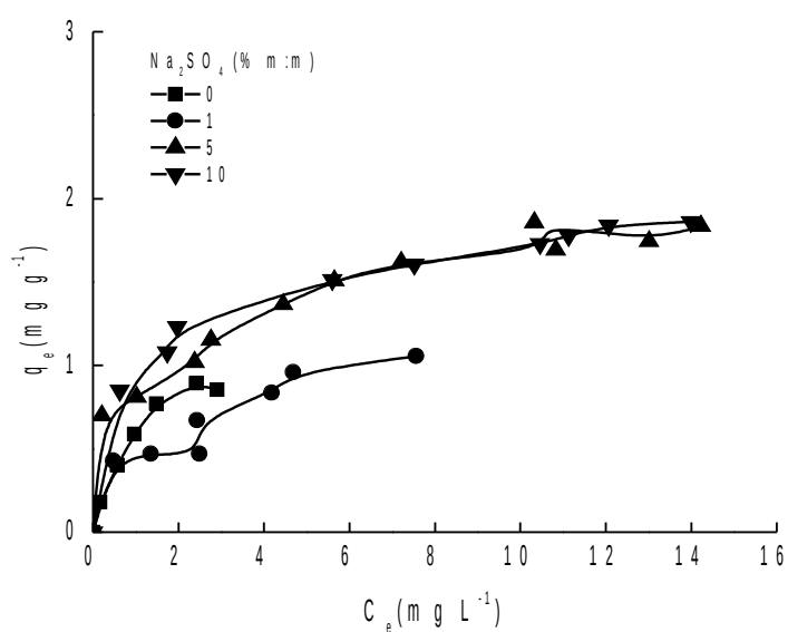
Figura 6. Isoterma de adsorção do RV sobre ZM-2 na presença de NaCl e Na 2 SO 4 (T=25 °C; pH =5)
