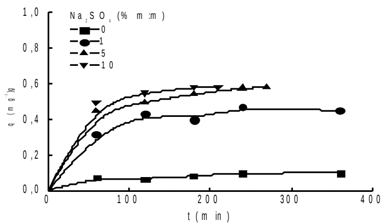
Figura 5. Efeito do tempo de agitação na remoção do RV sobre ZM-2 na presença de NaCl e \text{Na}_2\text{SO}_4 ( [\text{RV}] = 6 \text{ mg L}^{-1} ; T = 25 \text{ }^\circ\text{C} ; \text{pH} = 5 )
