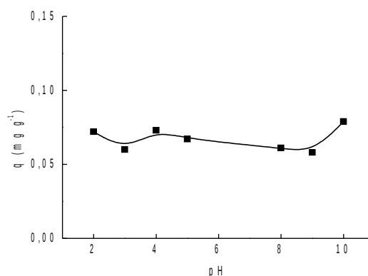
Figura 4. Influência do pH na adsorção do RV sobre ZM-2 ( [\text{RV}] = 2 \text{ mg L}^{-1} ; T = 25^\circ\text{C} ; t_{\text{agit}} = 360 \text{ min} )
