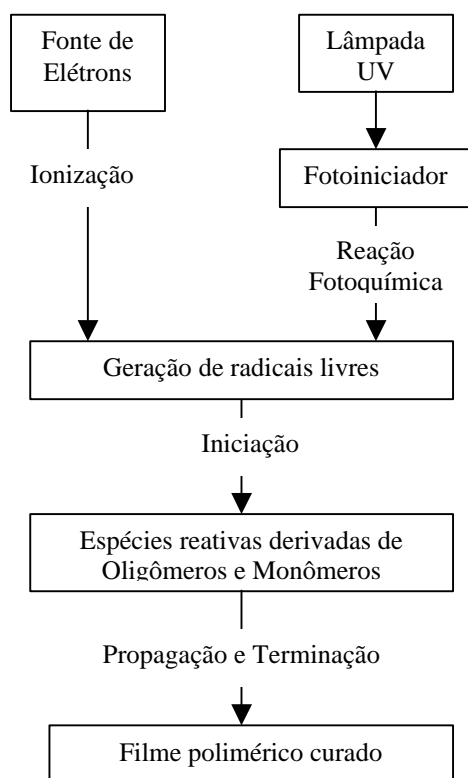
Figura 1. Etapas de Cura UV e EB.
