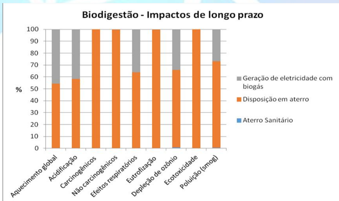
Figura 4. Resultado da ACV por categoria de impacto para biodigestão em longo prazo
