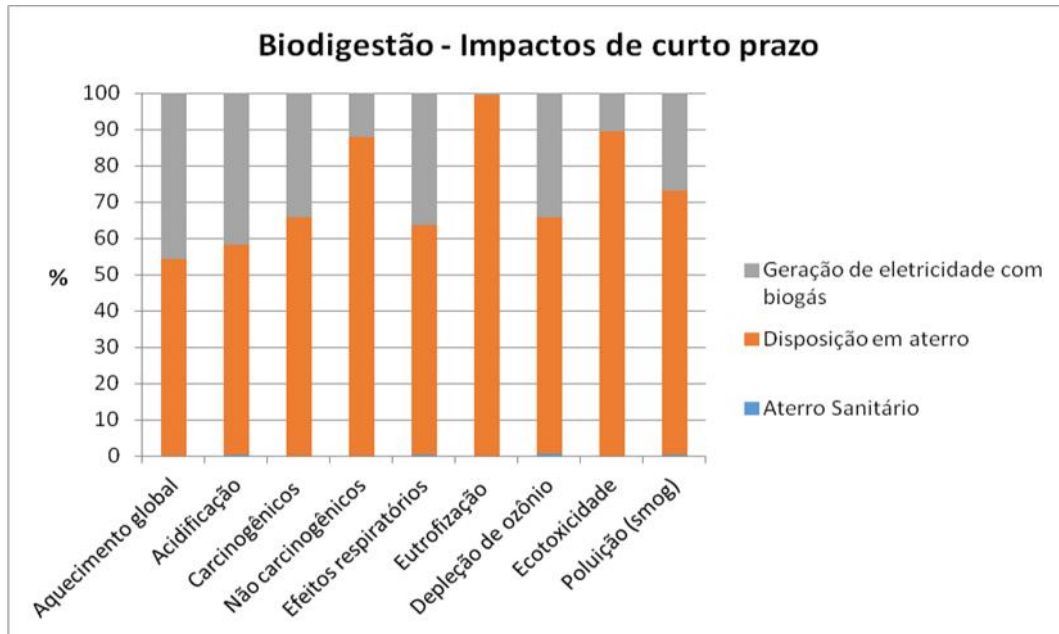
Figura 3. Resultados da ACV por categoria de impacto, para biodigestão em curto prazo.
