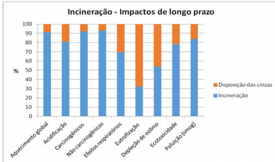
Figura 2. Resultado da ACV por categoria de impacto para incineração em longo prazo
