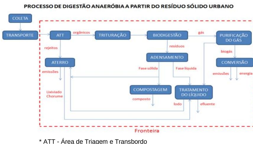
Figura 1. Fluxograma do processo e fronteira do estudo para biodigestão
