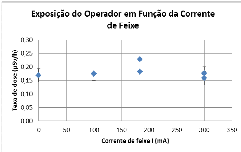
Figura 3: Gráfico da exposição do operador em função da corrente de feixe
