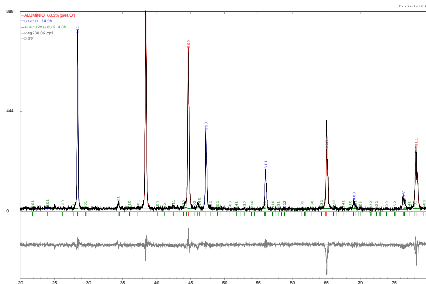
Figura 5. Espectro referente à análise por difração de raio X na liga 2 na condição como fabricada.
