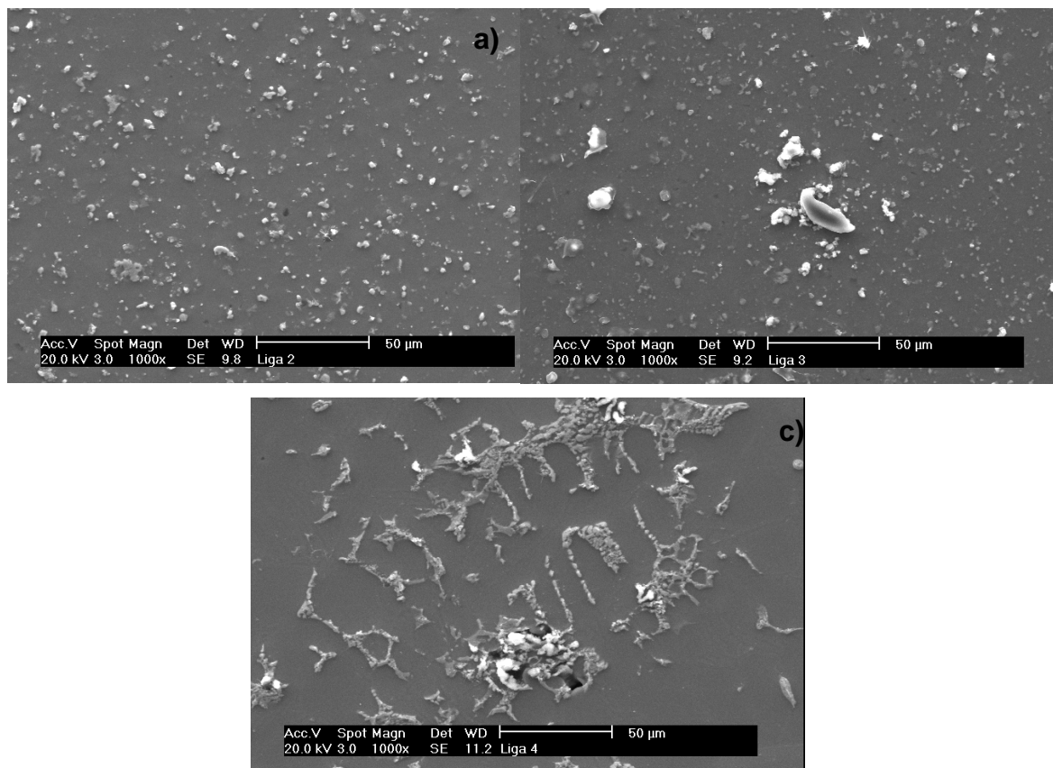
Figura 3. Micrografias obtidas em MEV das ligas produzida por conformação por spray (a) liga 2, (b) liga 3 e (c) liga 4.
