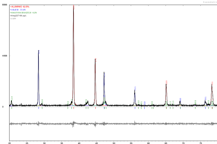
Figura 4. Espectro referente à análise por difração de raio X na liga 1 na condição como recebida.
