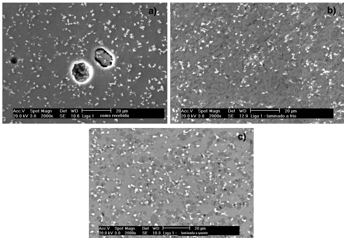
Figura 2. Micrografias obtidas em MEV de liga 1 experimental, produzida por conformação por spray (a) como recebida, (b) laminada a frio e (c) laminada a quente.
