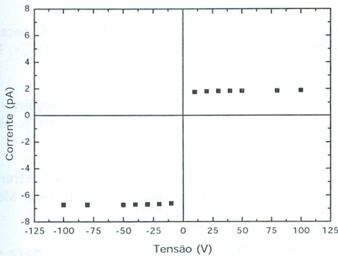
Figura 1: Curva de saturação da câmara de extrapolação, fonte de 90 Sr+ 90 Y (PTB), distância fonte-detector de 1,0 cm, distância intereletródica de 0,5mm e campo elétrico de 100V/mm
