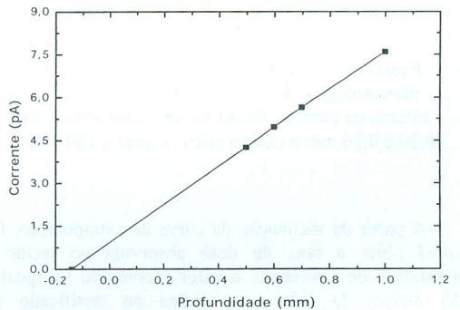
Figura 3: Curva de extrapolação para distâncias intereletródicas entre 0,5 e 1,0 mm, para a radiação beta de 90 Sr+ 90 Y, distância fonte-detector de 1,0 cm.
