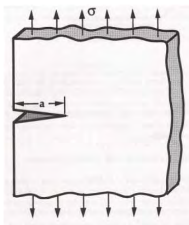
Figura 7 – Trinca de borda em uma chapa “infinita” sujeita a uma tensão de tração remota (7)
