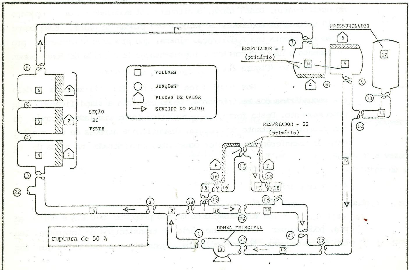
Figura 2 - Modelo do Circuito Experimental de Água
