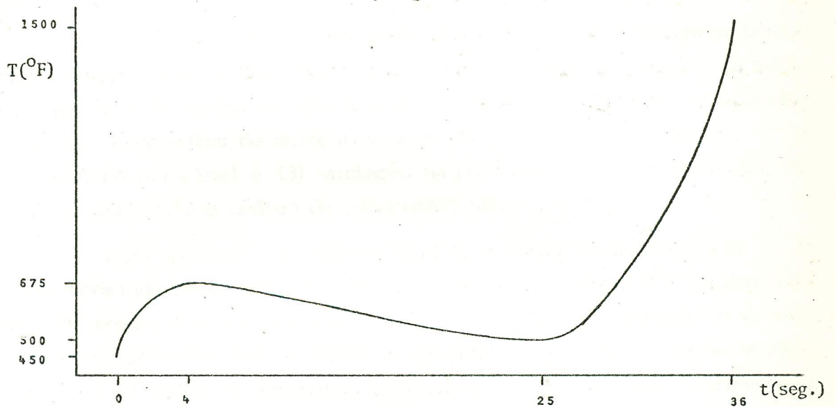
Figura 5 - Temperatura na placa 1
