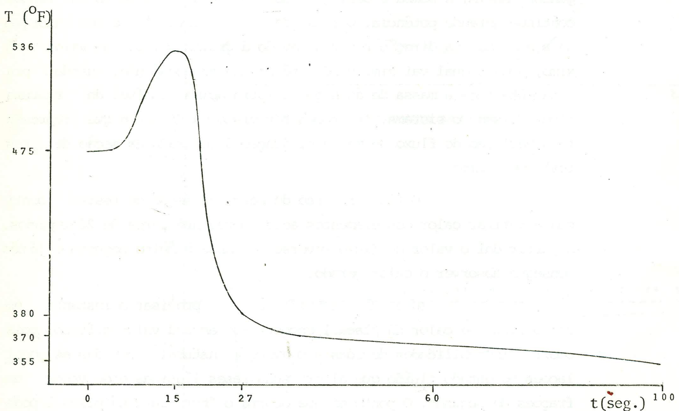
Figura 3 - Temperatura na placa 3
