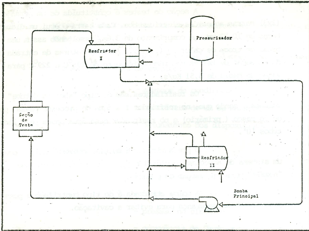
Figura 1 - Circuito Utilizado na Modelagem
