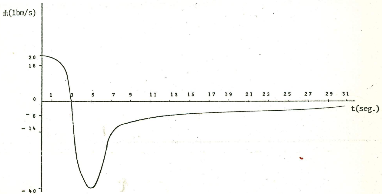
Figura 6 - Vazão de massa na seção de testes
