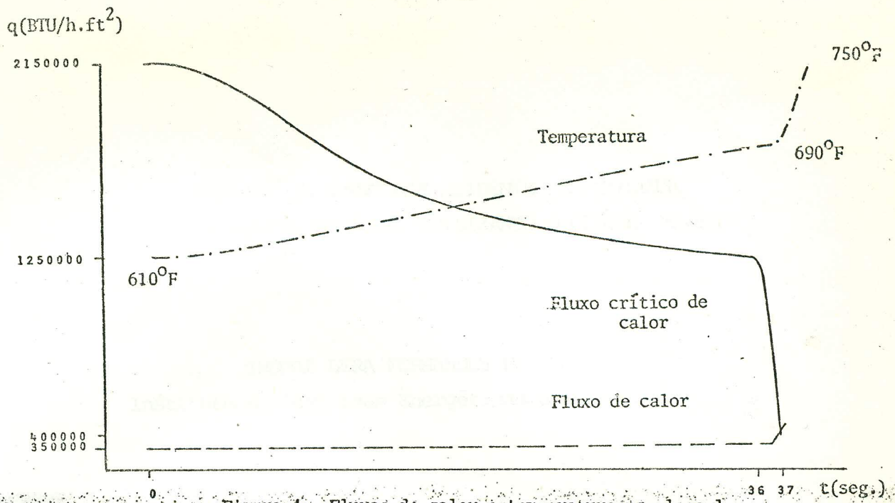
Figura 4 - Fluxos de calor e temperatura na placa 1
