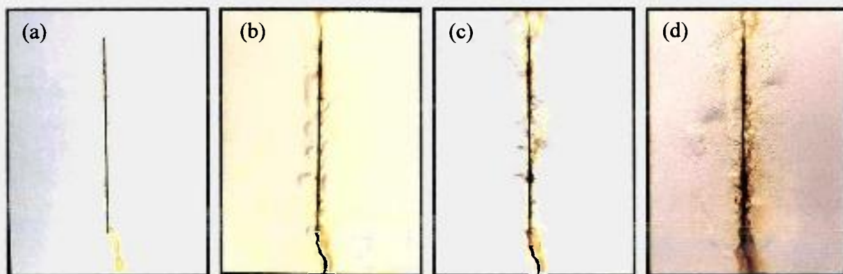
Figura 5.22 – Corpos-de-prova do sistema 2 após: (a) 164, (b) 832, (c) 1.000 e (d) 1.300 horas de ensaio Névoa Salina (ASTM B-117).
