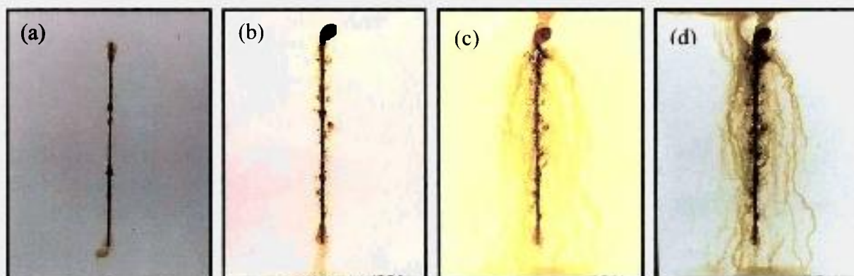
Figura 5.9 – Corpos-de-prova do sistema 4 após: (a) 259 horas de Prohesion e 192 horas de UVCON, (b) 380 horas de Prohesion e 392 horas de UVCON, (c) 764 horas de Prohesion e 807 horas de UVCON e (d) 1.000 horas de Prohesion e 1.000 horas de UVCON.
