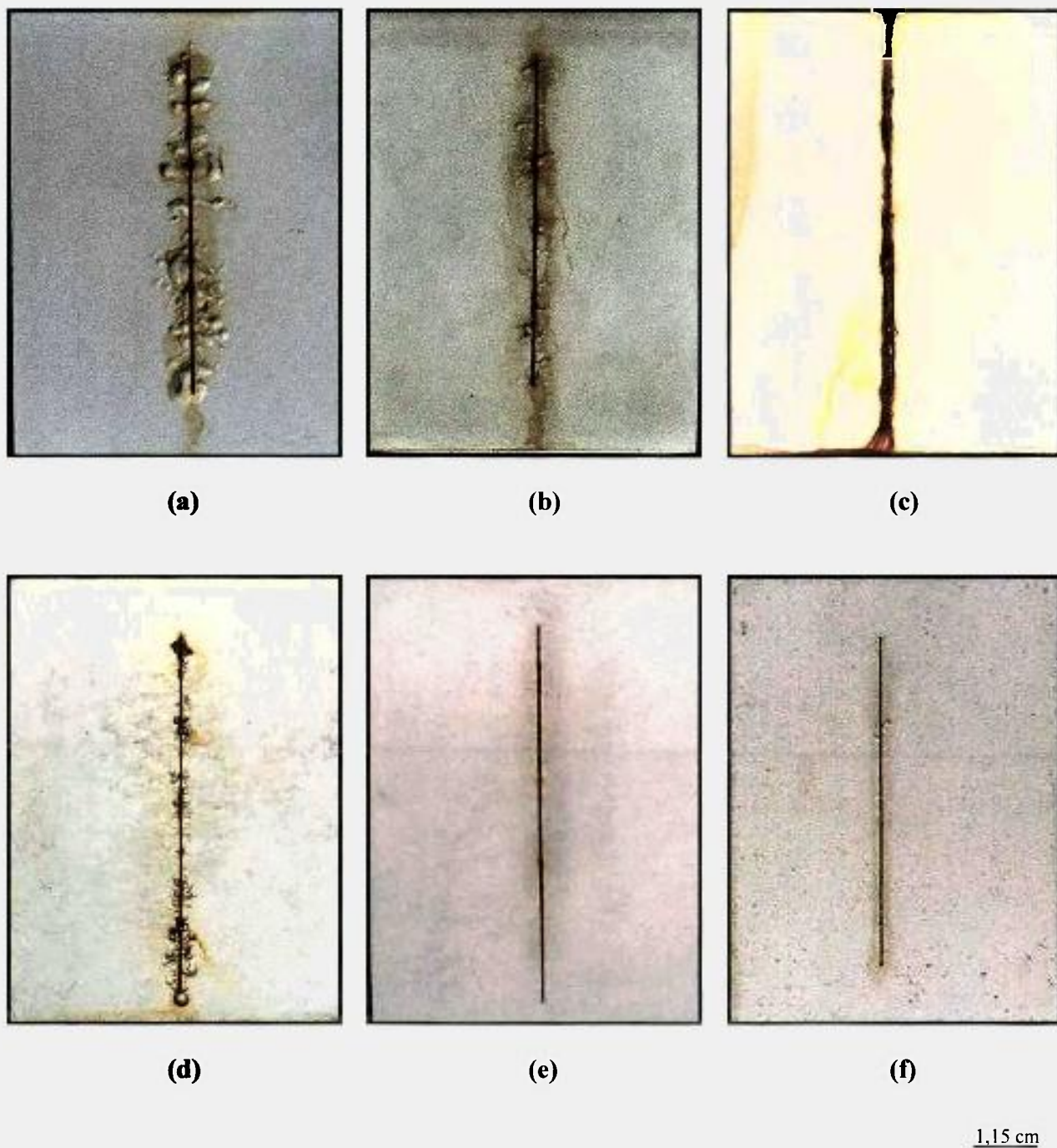
Figura 5.36 – Corpos-de-prova do sistema 5 após: (a) 2.000 horas de Prohesion, (b) 1.000 horas de Prohesion alternadas com 1.000 horas de UVCON, (c) 832 horas de ASTM B-117, (d) 2.000 horas de Prochuva, (e) 1.000 horas de Prochuva alternadas com 1.000 horas de UVCON e (f) 2 anos e meio de exposição ao intemperismo natural.
