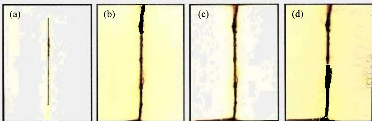
Figura 5.21 – Corpos-de-prova do sistema 1 após: (a) 164, (b) 832, (c) 1.000 e (d) 1.300 horas de ensaio Névoa Salina (ASTM B-117).
