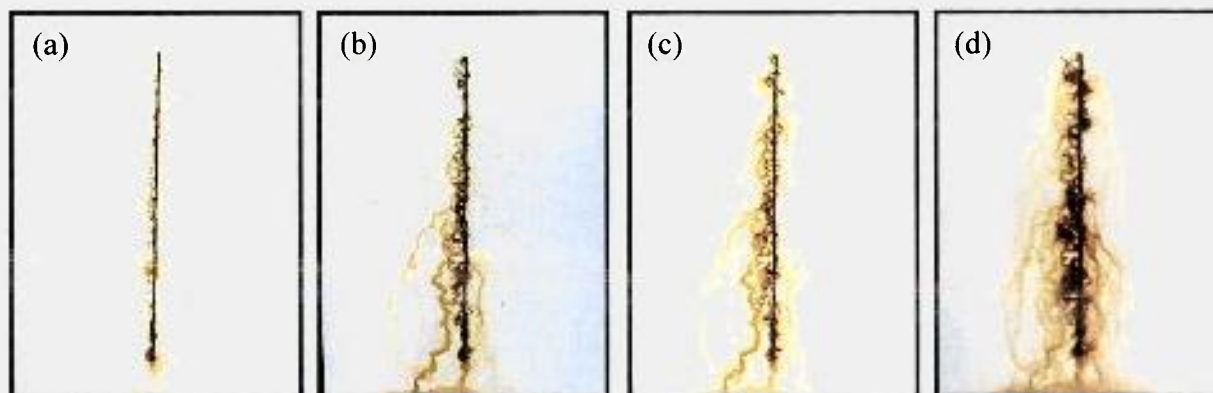
Figura 5.19 – Corpos-de-prova do sistema 4 após: (a) 232 horas de Prohchuva e 188 horas de UVCON, (b) 371 horas de Prohchuva e 380 horas de UVCON, (c) 558 horas de Prohchuva e 521 horas de UVCON e (d) 1.000 horas de Prohchuva e 1.000 horas de UVCON.
