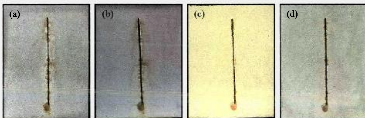
Figura 5.7 – Corpos-de-prova do sistema 2 após: (a) 259 horas de Prohesion e 192 horas de UVCON, (b) 380 horas de Prohesion e 392 horas de UVCON, (c) 764 horas de Prohesion e 807 horas de UVCON e (d) 1000 horas de Prohesion e 1000 horas de UVCON.
