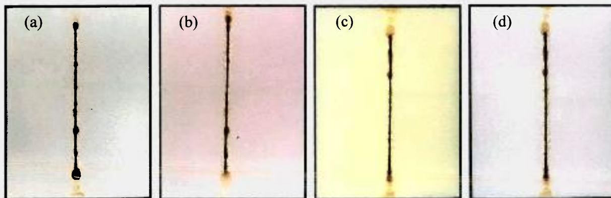
Figura 5.4 – Corpos-de-prova do sistema 4 após: (a) 570, (b) 1.032, (c) 1.439 e (d) 2.000 horas de ensaio Prohesion.
