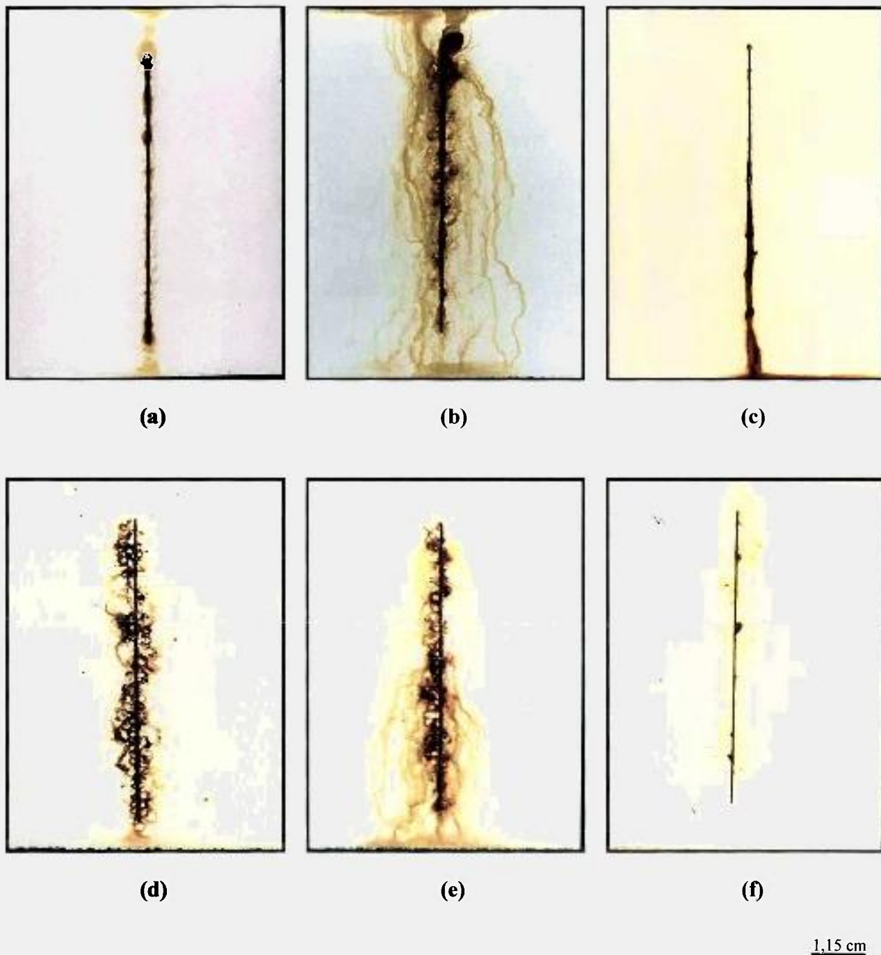
Figura 5.35 – Corpos-de-prova do sistema 4 após: (a) 2.000 horas de Prohesion, (b) 1.000 horas de Prohesion alternadas com 1.000 horas de UVCON, (c) 832 horas de ASTM B-117, (d) 2.000 horas de Prochuva, (e) 1.000 horas de Prochuva alternadas com 1.000 horas de UVCON e (f) 2 anos e meio de exposição ao intemperismo natural.
