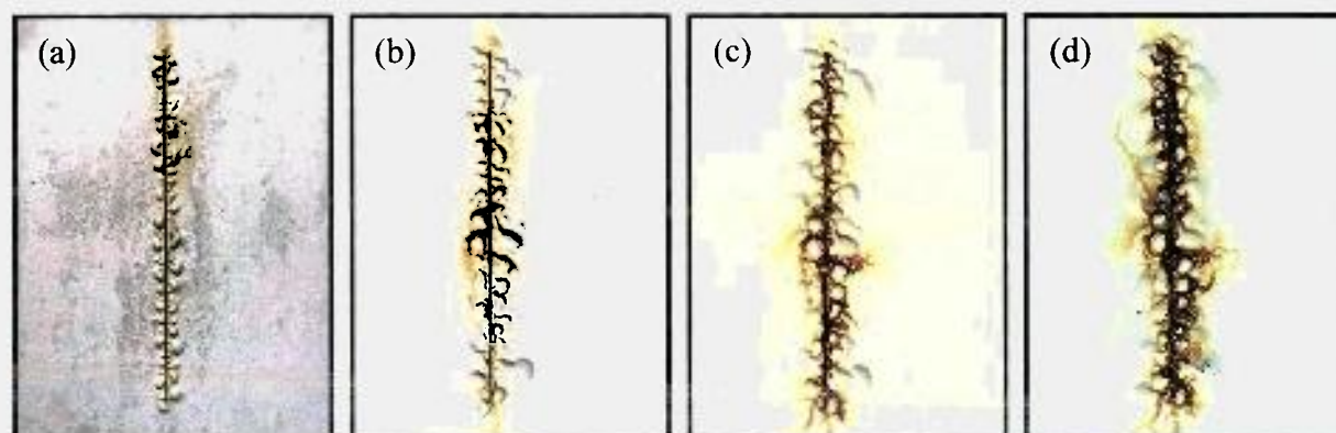
Figura 5.13 – Corpos-de-prova do sistema 3 após: (a) 635, (b) 1.080, (c) 1.535 e (d) 2.000 horas de ensaio Prohchuva.
