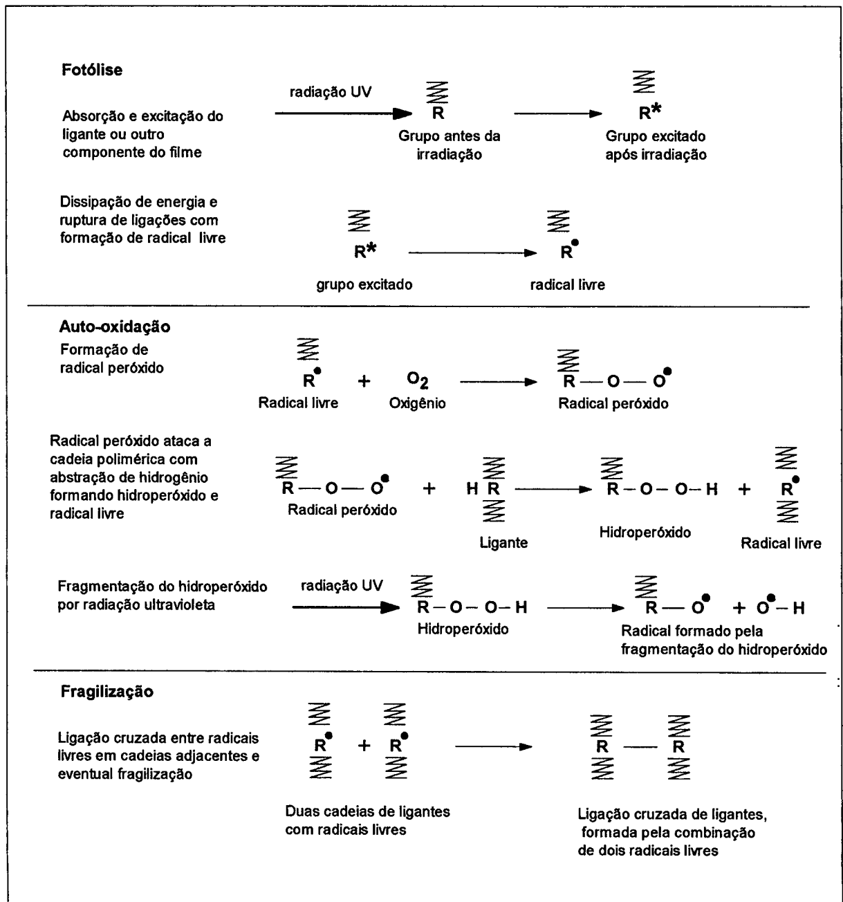
Figura 2.4 – Representação esquemática da degradação de revestimentos orgânicos por radiação UV[32].
