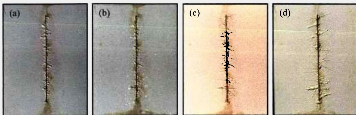
Figura 5.2 – Corpos-de-prova do sistema 2 após: (a) 570, (b) 1.032, (c) 1.439 e (d) 2.000 horas de ensaio Prohesion.
