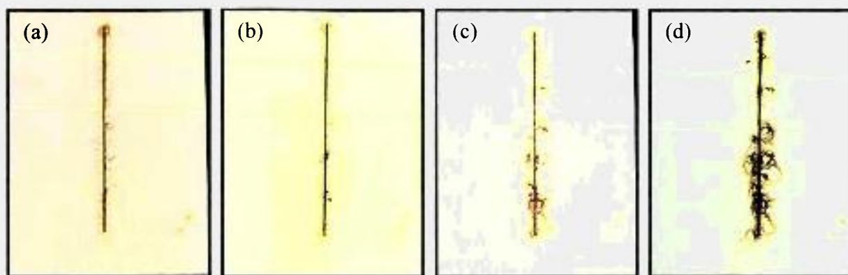
Figura 5.11 – Corpos-de-prova do sistema 1 após: (a) 635, (b) 1.080, (c) 1.535 e (d) 2.000 horas de ensaio Prohchuva.
