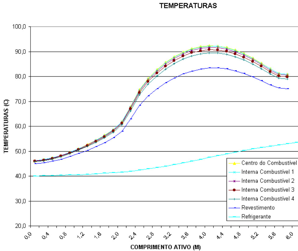
Figura 3. Temperaturas ao Longo do Comprimento Ativo.
