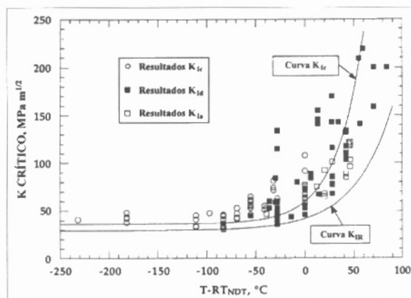
Figura 2 – Envoltórias K_{IC} e K_{IR}
