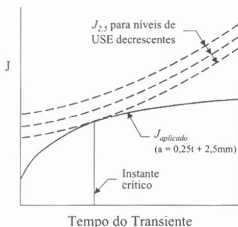
Figura 7 – USE que satisfaz critério de aceitação I
