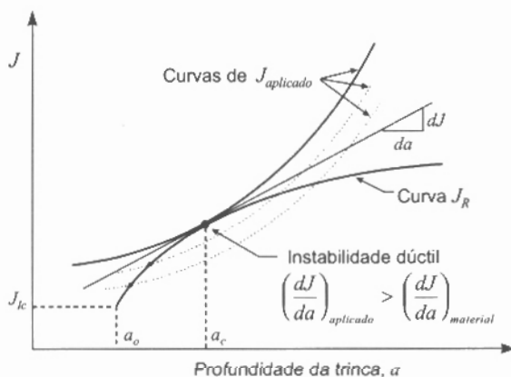
Figura 6 – Representação gráfica da instabilidade dúctil
