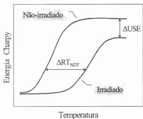
Figura 1 – Medidas de redução da tenacidade
