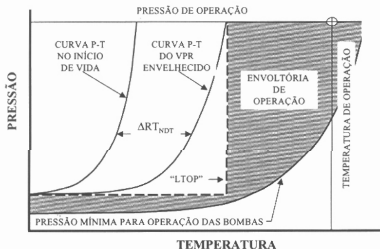
Figura 3 – Efeito da fragilização por irradiação nas curvas-limite P-T
