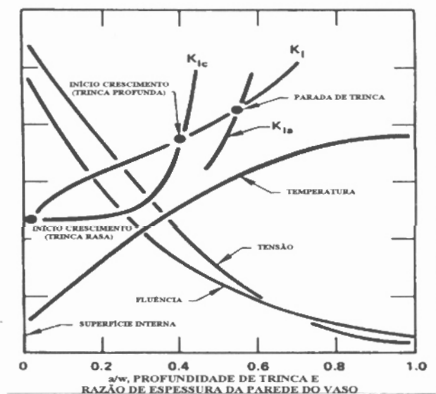
Figura 5 – Comportamento das diversas variáveis num dado instante do transiente de PTS
