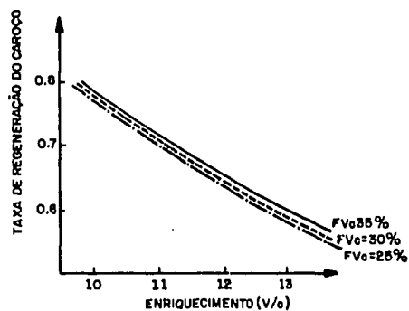
FIGURA ( 7 ): TAXA DE REGENERAÇÃO DO CAROÇO X ENRIQUECIMENTO DO GCFR
