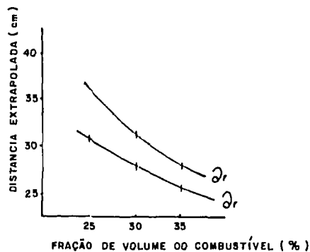
FIGURA (10): Distância extrapolada x fração de volume do combustível do GCFR
