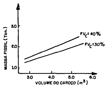
FIGURA (16): MASSA FISSIL X VOLUME DO CAROÇO DO LMFBR
