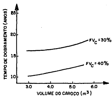
FIGURA (17): TEMPO DE DOBRAMENTO X VOLUME DO CAROÇO DO LMFBR
