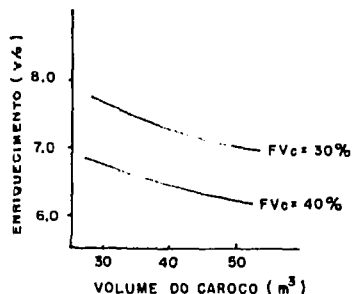
FIGURA (12): Enriquecimento x volume do caroço do LMFBR
