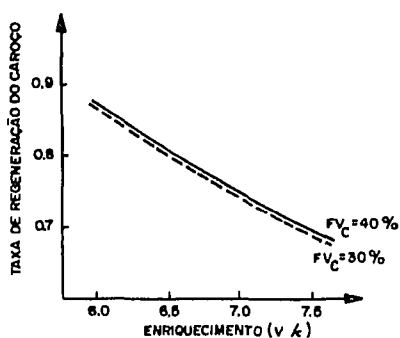
FIGURA (15): TAXA DE REGENERAÇÃO DO CAROÇO X ENRIQUECIMENTO DO LMFBR
