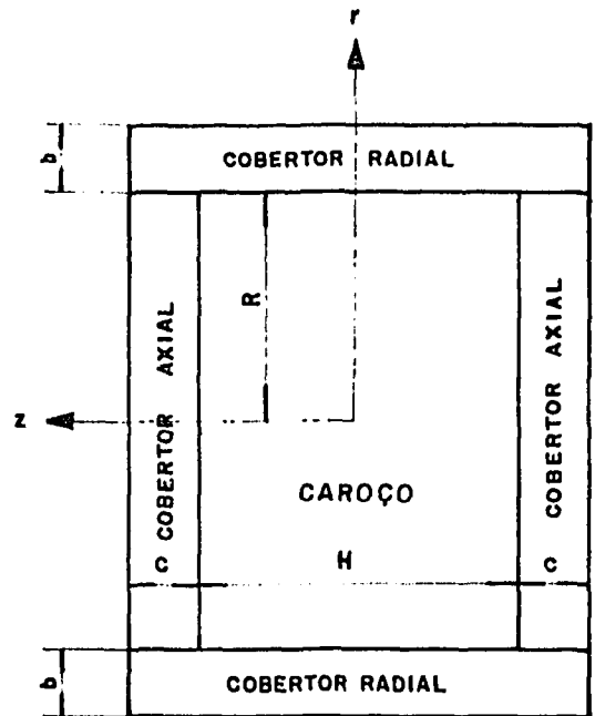
Figura (2): Seção Axial
