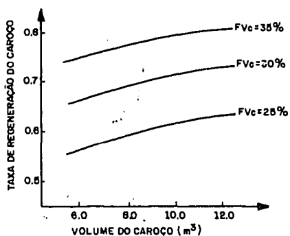
FIGURA ( 5 ): TAXA DE REGENERAÇÃO DO CAROÇO X VOLUME DO CAROÇO DO GCFR
