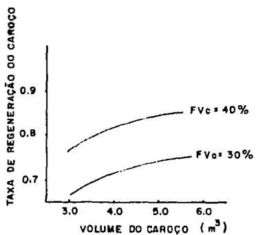
FIGURA (13): Taxa de regeneração do caroço x volume do caroço do LMFBR
