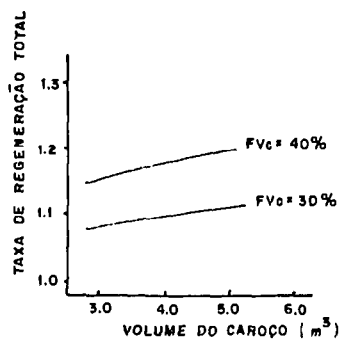
FIGURA (14): Taxa de regeneração total x volume do caroço do LMFBR
