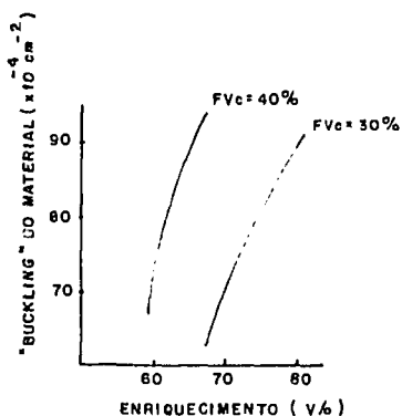
FIGURA (11): "BUCKLING" do material x enriquecimento de LMFBR
