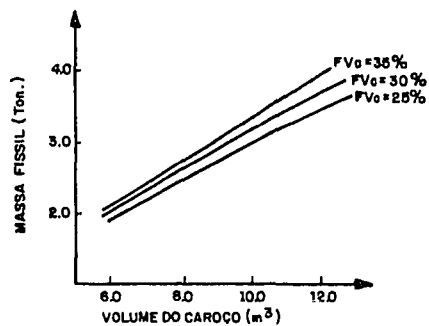
FIGURA ( 8 ): MASSA FÍSSIL X VOLUME DO CAROÇO DO GCFR
