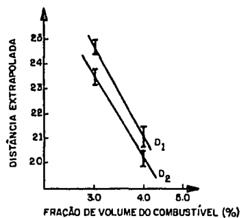
FIGURA (18): DISTÂNCIA EXTRAPOLADA X FRAÇÃO DE VOLUME DO COMBUSTÍVEL DO LMFBR
