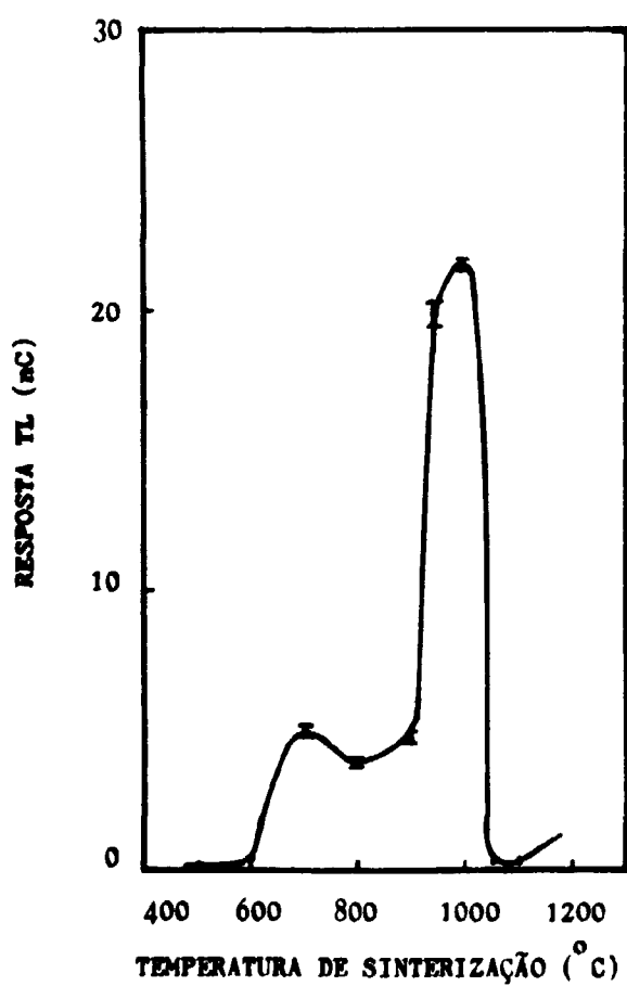
Figura 5: Resposta TL do \text{MgB}_4\text{O}_7:\text{Dy} em função da temperatura de sinterização ( t = 1\text{h} )
