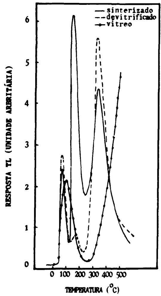
Figura 7: Curva de emissão TL do \text{CaB}_4\text{O}_7:\text{Dy}
