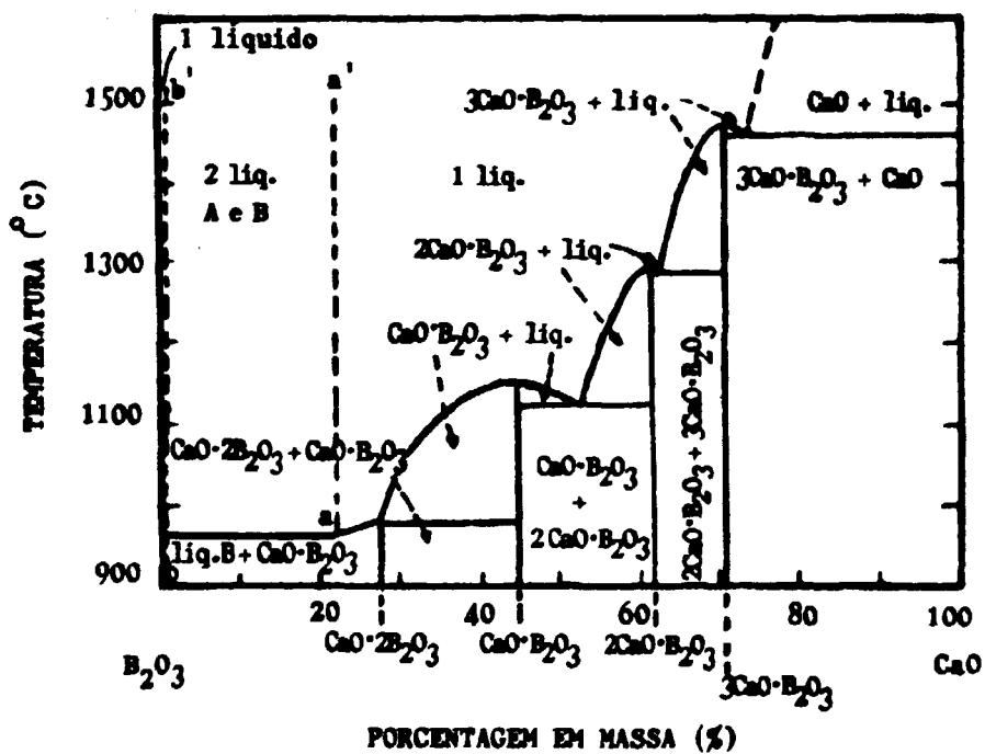
Figura 2: Diagrama de fases do sistema B_2O_3 - CaO
