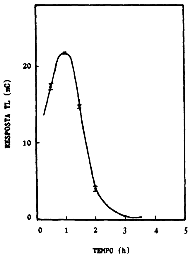
Figura 6: Resposta TL do \text{MgB}_4\text{O}_7:\text{Dy} em função do tempo de sinterização ( T = 1000^\circ\text{C} )
