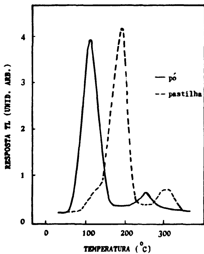
Figura 3: Curva de emissão TL do \text{MgB}_4\text{O}_7:\text{Dy}
