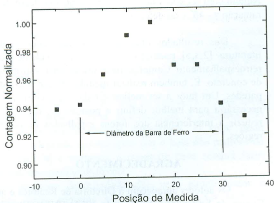
Figura 6 – Medidas para avaliar o diâmetro da barra de ferro. Ângulo com relação a horizontal: incidência do feixe de radiação \gamma - 45^\circ e do detector - 90^\circ .
