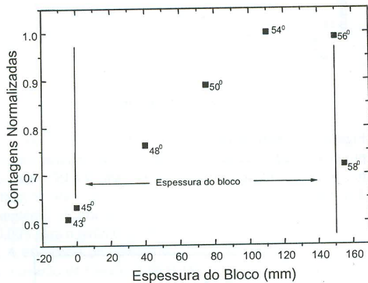
Figura 5 – Medidas para avaliar a espessura do bloco de concreto. O ângulo de incidência do feixe de radiação \gamma com relação a horizontal é apresentado junto aos pontos.
