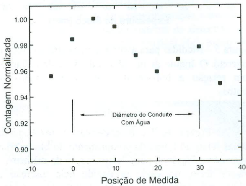
Figura 8 – Medidas para avaliar a resposta do retroespalhamento em água no diâmetro do condute. Ângulo com relação a horizontal: incidência do feixe de radiação \gamma - 45^\circ e do detector - 90^\circ .
