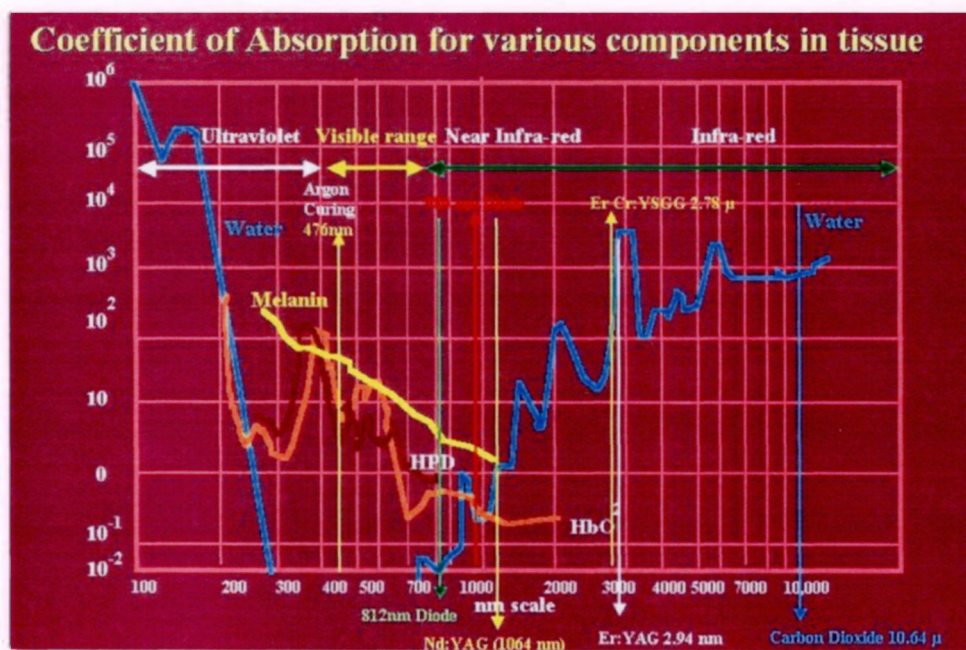
“FIGURA 03. Espectro de absorção dos principais cromóforos dos tecidos biológicos”
