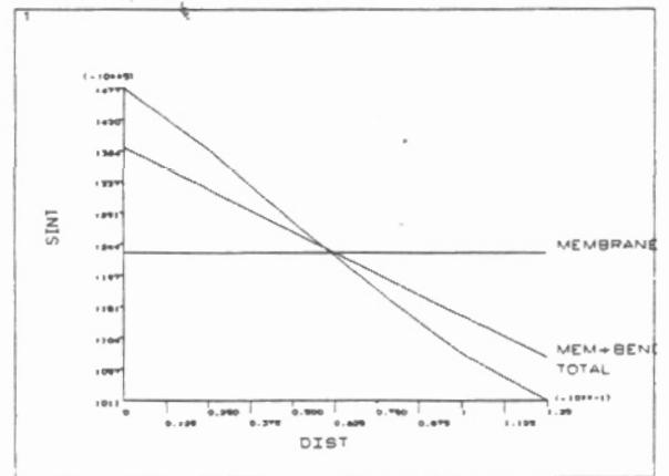
figura 15 -- Seção 4: Contribuição nula de SX, SXY, SYZ e SXZ para a flexão
