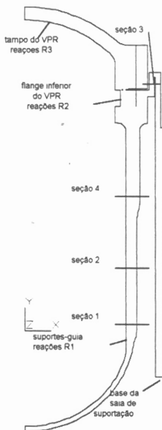
figura 1 - Modelo do VPR
