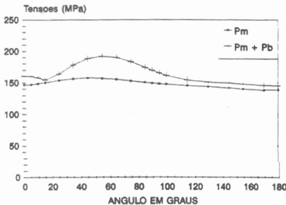
fig. 7 - Tensões SI linearizadas na seção 2
