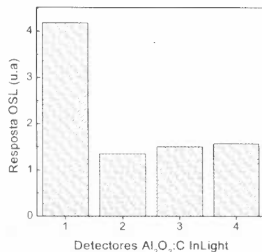
Figura 2: 3 - Resposta OSL dos detectores \text{Al}_2\text{O}_3:\text{C} InLight após exposição à RUV durante 2 min de soldagem elétrica.
