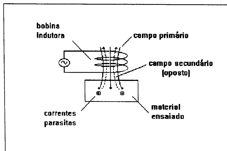
Figura 1. Geração de Correntes Parasitas num material
