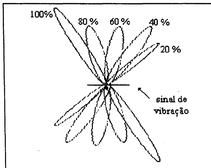
Figura 3. Figuras de Lissajous para um tubo-padrão de referência ASME
