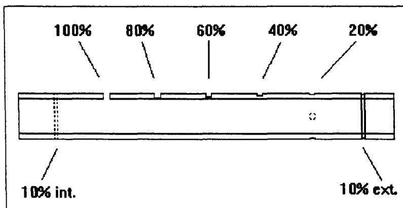
Figura 2. Tubo de referência ou padrão de calibração
