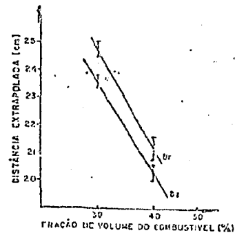
Figura (18) : Distância extrapolada x fração de volume do combustível do IMFBR
