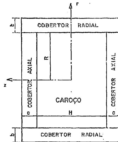
Figura (2) : Secção Axial
