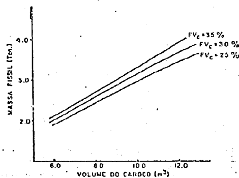
Figura (8) : Massa físsil x volume do caroço do GCFR
