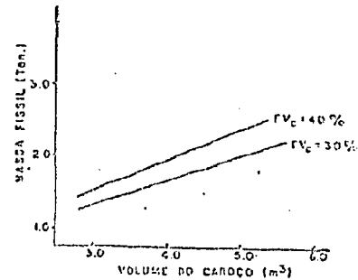
Figura (16) : Massa físsil x volume do caroço do IMFBR
