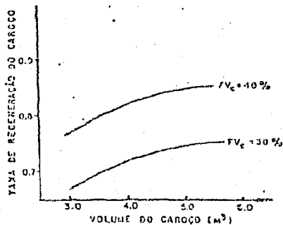
Figura (13) : Taxa de regeneração do caroço x volume do caroço do IMFBR
