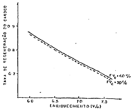
Figura (15) : Taxa de regeneração do caroço x enriquecimento do IMFBR
