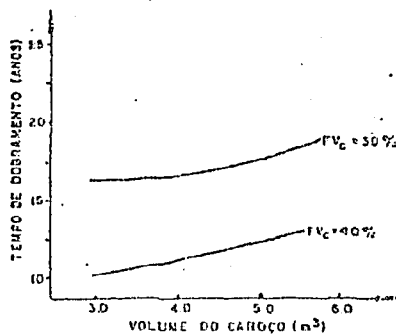
Figura (17) : Tempo de dobramento x volume do caroço do IMFBR
