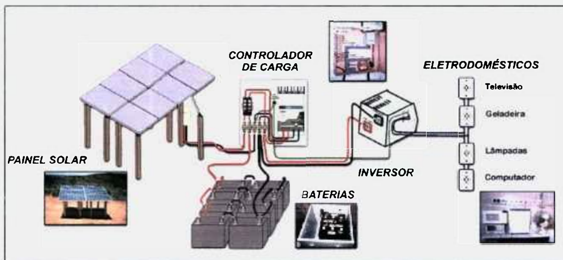
FIGURA 3.1 - Sistema fotovoltaico de geração de energia elétrica
