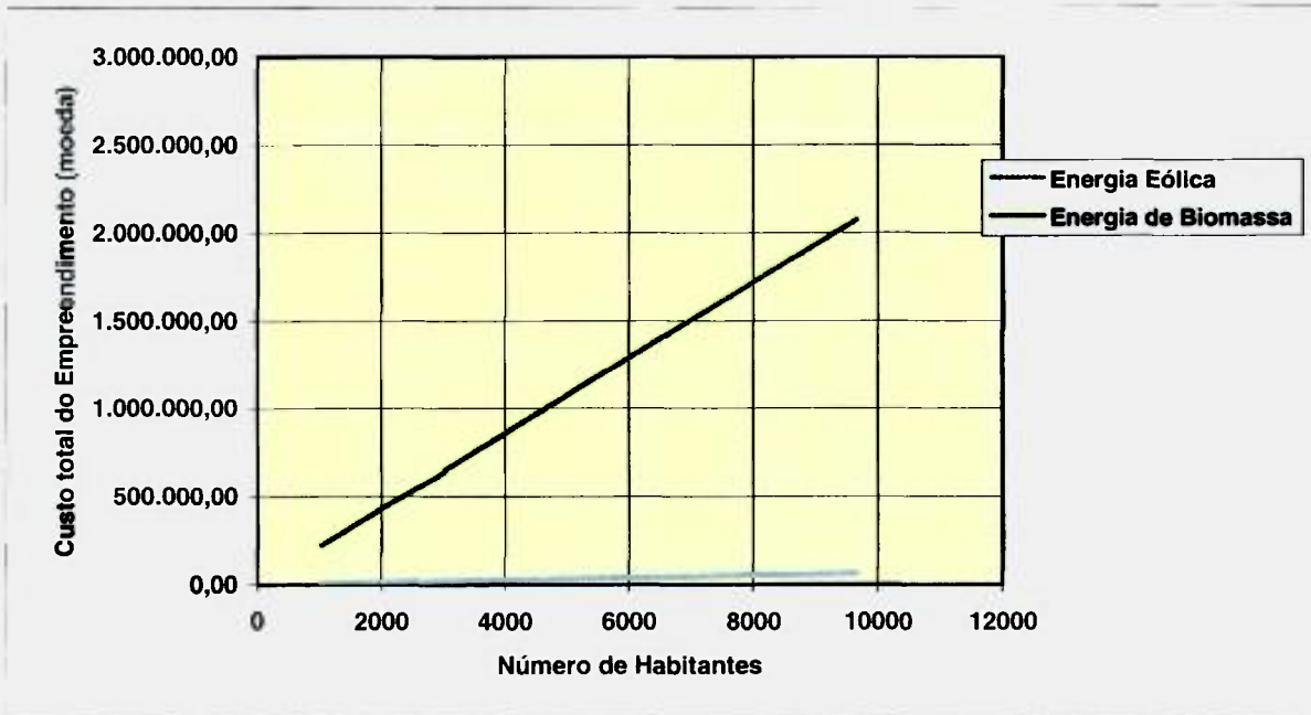
FIGURA 7.5 - Comparação dos custos totais dos empreendimentos de biomassa e eólico, nos tempos de vida correspondentes, em função de número de habitantes
