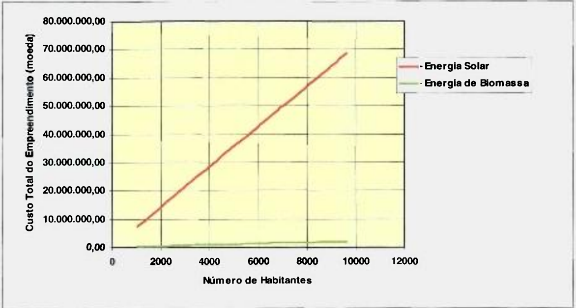
FIGURA 7.4 - Comparação dos custos totais dos empreendimentos solar e de biomassa, nos tempos de vida correspondentes, em função de número de habitantes
