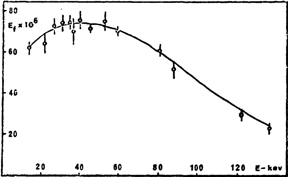
EFICIÊNCIA TOTAL DE DETECÇÃO X ENERGIA GAMA
