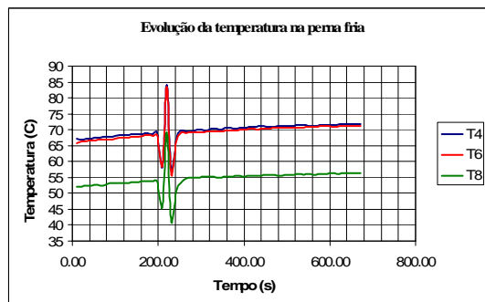
FIGURA 4. Evolução da temperatura na perna fria
