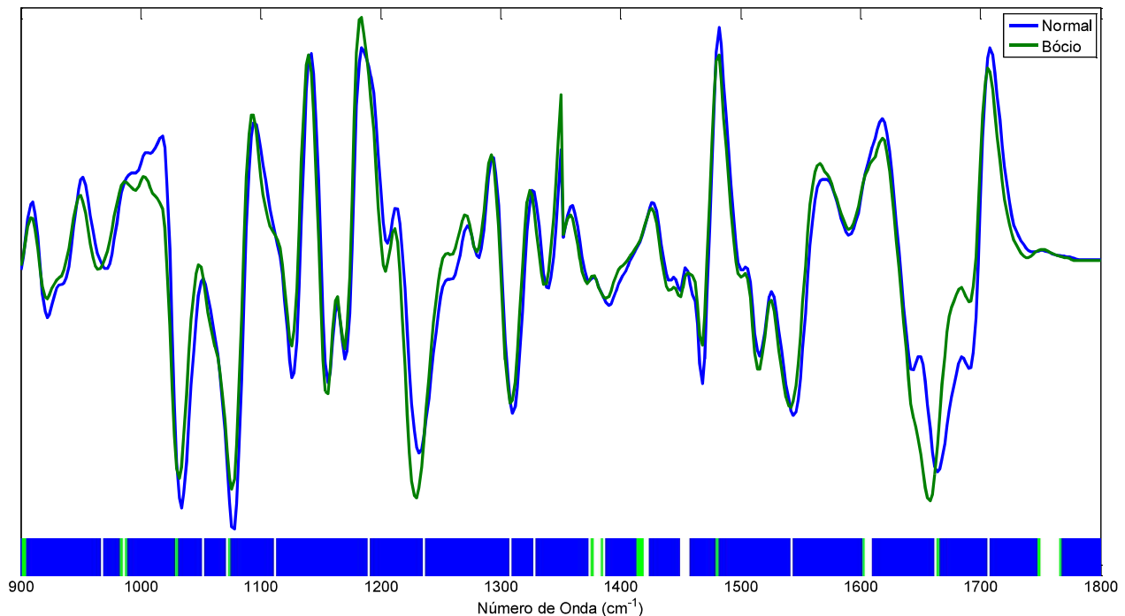
Figura 1: Espectros médios de colóides provenientes de tecidos normais e com bócio nodular. A barra de cor representa o resultado do t test . Regiões em azul são estatisticamente significante considerando valor de p menor que 0,01. Regiões em verde são estatisticamente significante considerando valor de p menor que 0,05.
