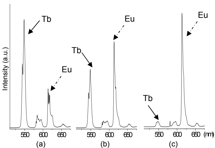
Figura 2. Espectros de emissão (a 298K) do filme PMMA dopado com \text{Eu}(\text{tta})_3 \cdot 2\text{H}_2\text{O} e \text{Tb}(\text{acac})_3 \cdot 3\text{H}_2\text{O} , com excitações a: a) 315 nm, b) 330 nm e c) 367 nm.
