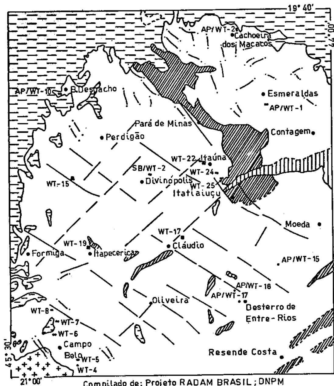
FIGURA 2 - ESBOÇO GEOLÓGICO DA ÁREA INVESTIGADA
