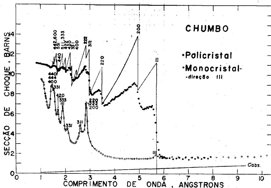
Figura 1 - A curva teórica é a de seção de choque de espalhamento coerente elástico a 0° K. As curvas experimentais foram obtidas à temperatura ambiente. Os números se referem a índices de Miller hkl de planos de distância interplanar d_{hkl} .
