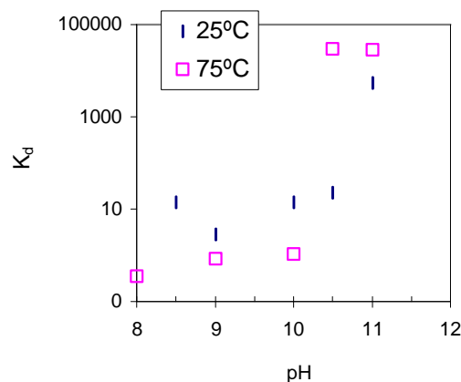
Figura 1. Variação de K_d do Eu^{3+} nos Diferentes Materiais de Ferro formados em Diferentes pH de Precipitação.
