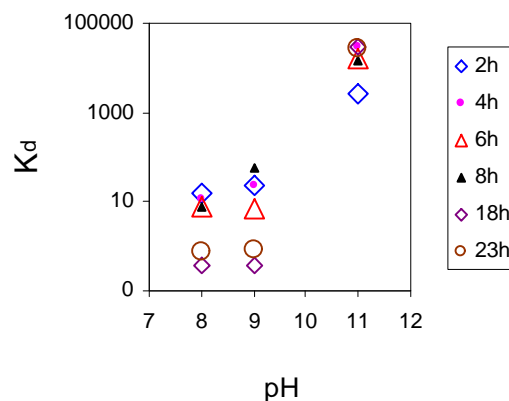
Figura 2. Variação de K_d do Eu^{3+} nos Compostos de Ferro formados em pH Diferentes e Secos por Tempos Diferentes, à Temperatura Ambiente.
