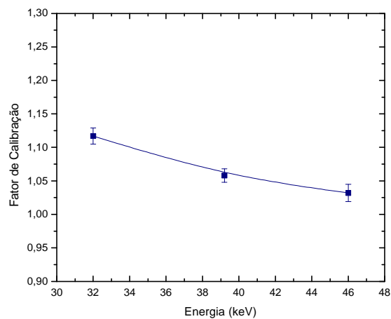
Figura 1. Dependência Energética da Câmara de CT nas Qualidades de Radiodiagnóstico, Feixes Diretos, Equipamento Medcor Mövek Röntgengyara .
