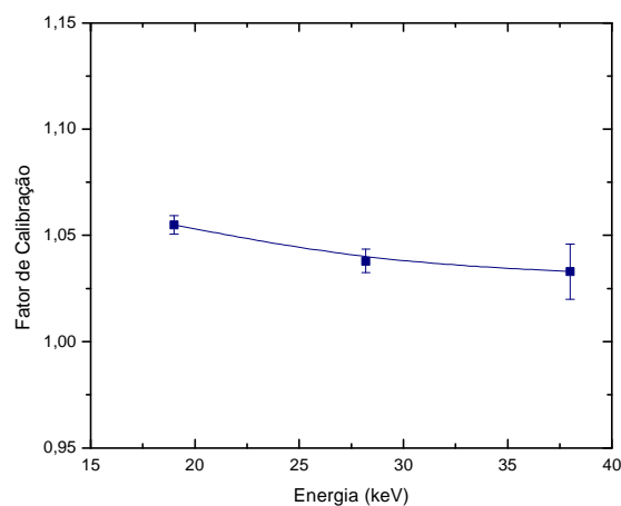
Figura 3. Dependência Energética da Câmara de CT nas Qualidades de Radiodiagnóstico, Equipamento Rigaku Denki .
