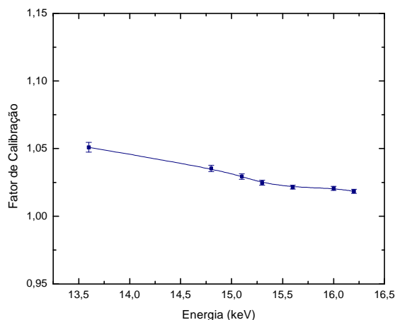
Figura 4. Dependência Energética da Câmara de CT nas Qualidades de Mamografia, Feixes de Entrada, Equipamento Rigaku Denki .
