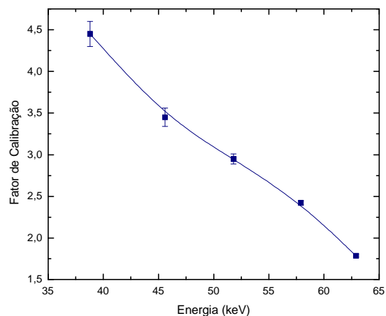
Figura 2. Dependência Energética da Câmara de CT nas Qualidades de Radiodiagnóstico, Feixes Atenuados, Equipamento Medcor Mövek Röntgengyara .
