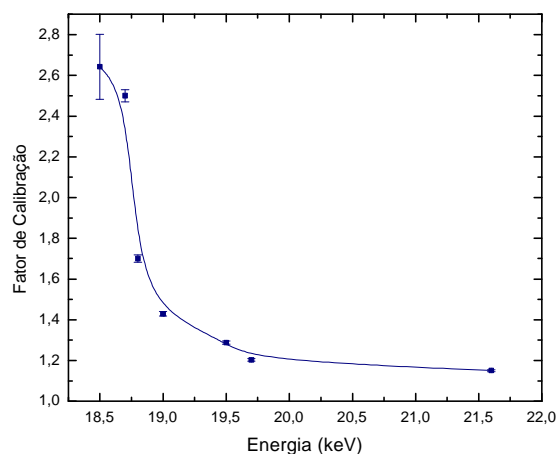
Figura 5. Dependência Energética da Câmara de CT nas Qualidades de Mamografia, Feixes de Saída, Equipamento Rigaku Denki .
