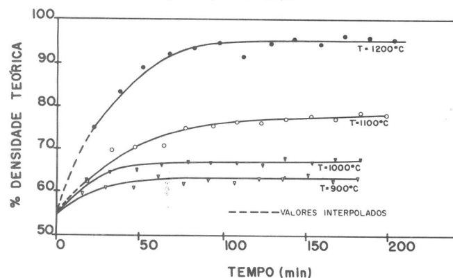
Figura 7 — Densidades típicas, em % D.T., observadas durante a sinterização, em função do tempo. Os valores de I correspondentes ao início das curvas (após os valores interpolados na figura), foram obtidos aplicando a expressão (C).
