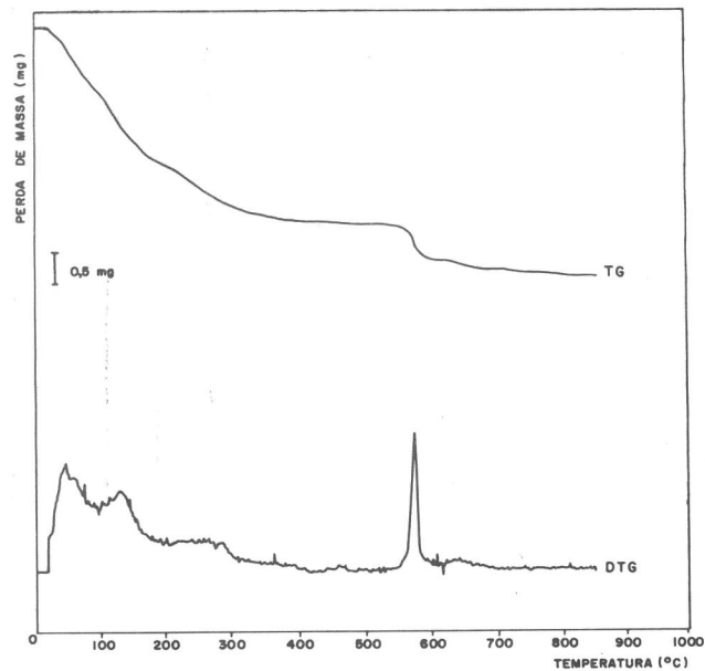
Figura 3 — Curvas TG e DTG da decomposição térmica do diuranato de amônio.
