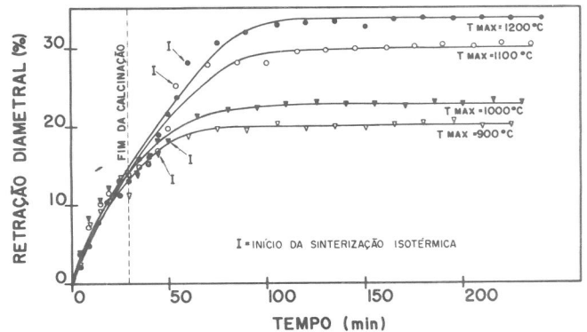
Figura 4 — Retrações diametrais típicas observadas durante a calcinação e sinterização em função do tempo. Sinterização isotérmica desenvolvida em 3 horas; curvas ajustadas para os dados experimentais plotados.
