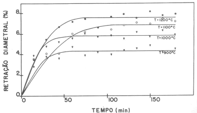
Figura 5 — Retrações diametrais típicas de microesferas de U_3O_8 durante sinterização isotérmica, em função do tempo, até 3 horas; curvas ajustadas (SAS) para os dados experimentais plotados.
