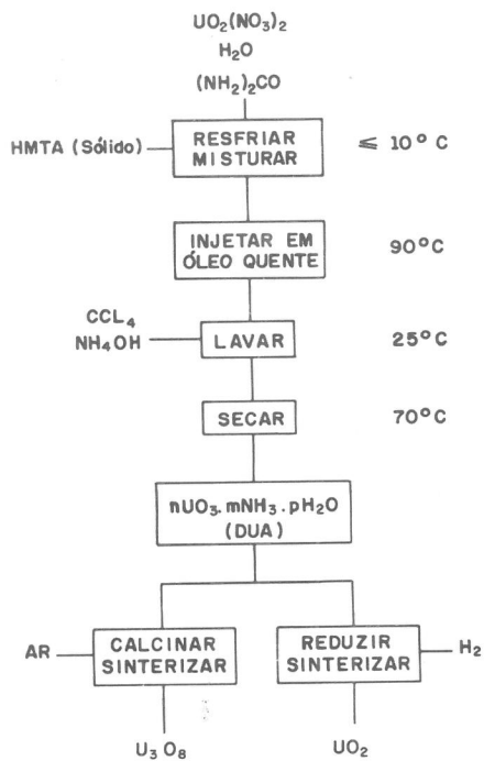
Figura 1 — Fluxograma do processo-H para fabricação de microesferas de UO_2 e U_3O_8 .
