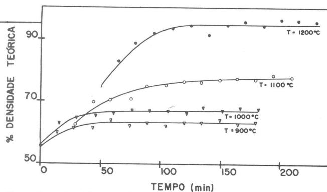
Figura 6 — Densidades típicas, em % D.T., observadas durante a sinterização em função do tempo. Os valores de I correspondentes ao início das curvas foram calculados pela expressão (A).
