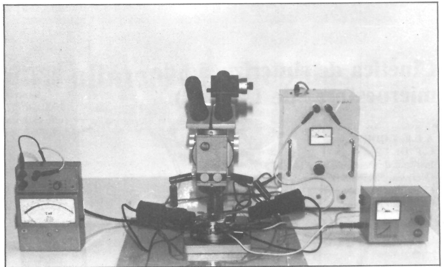
Figura 2 — Arranjo experimental utilizado.
