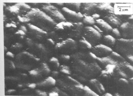
Figura 9 — Micrografia eletrônica de uma microesfera sinterizada a 1200°C.
