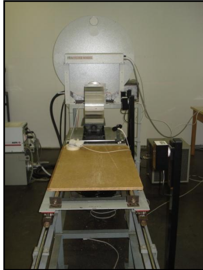
Figura 2: Sistema de radiação X, Pantak Isovolt HS 160 I
