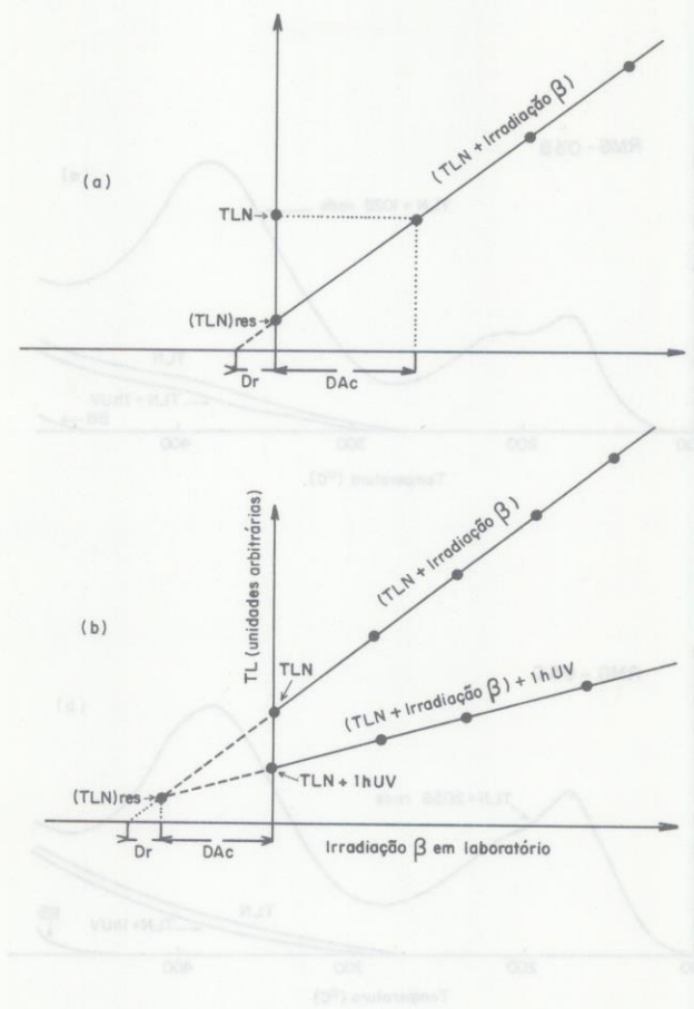
FIG. 7 - DETERMINAÇÃO DAS DOSES ACUMULADAS ( D_{ac} ) PELO MÉTODO DAS "DOSES ADITIVAS" (VER TEXTO)
