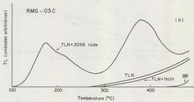
FIG. 8 - ESPECTROS DA TL DAS AMOSTRAS RMG - 03 B E RMG-03 C. NOTAR QUE (1) O PICO DE 380°C NÃO É AINDA APARENTE NAS CURVAS DA TLN, MAS MOSTRA-SE BEM DESENVOLVIDO APÓS UMA IRRADIAÇÃO BETA DE 1 A 2 KRADS EM LABORATÓRIO; E (2) UMA EXPOSIÇÃO DE 1h SOB LAMPADA UV PROVOCA UMA REDUÇÃO NA INTENSIDADE DO SINAL DA TLN EM TODAS AS TEMPERATURAS. A CURVA BB ("BLACK BODY") REPRESENTA A LUZ EMITIDA PELO FORNO DE TL À ALTAS TEMPERATURAS.
